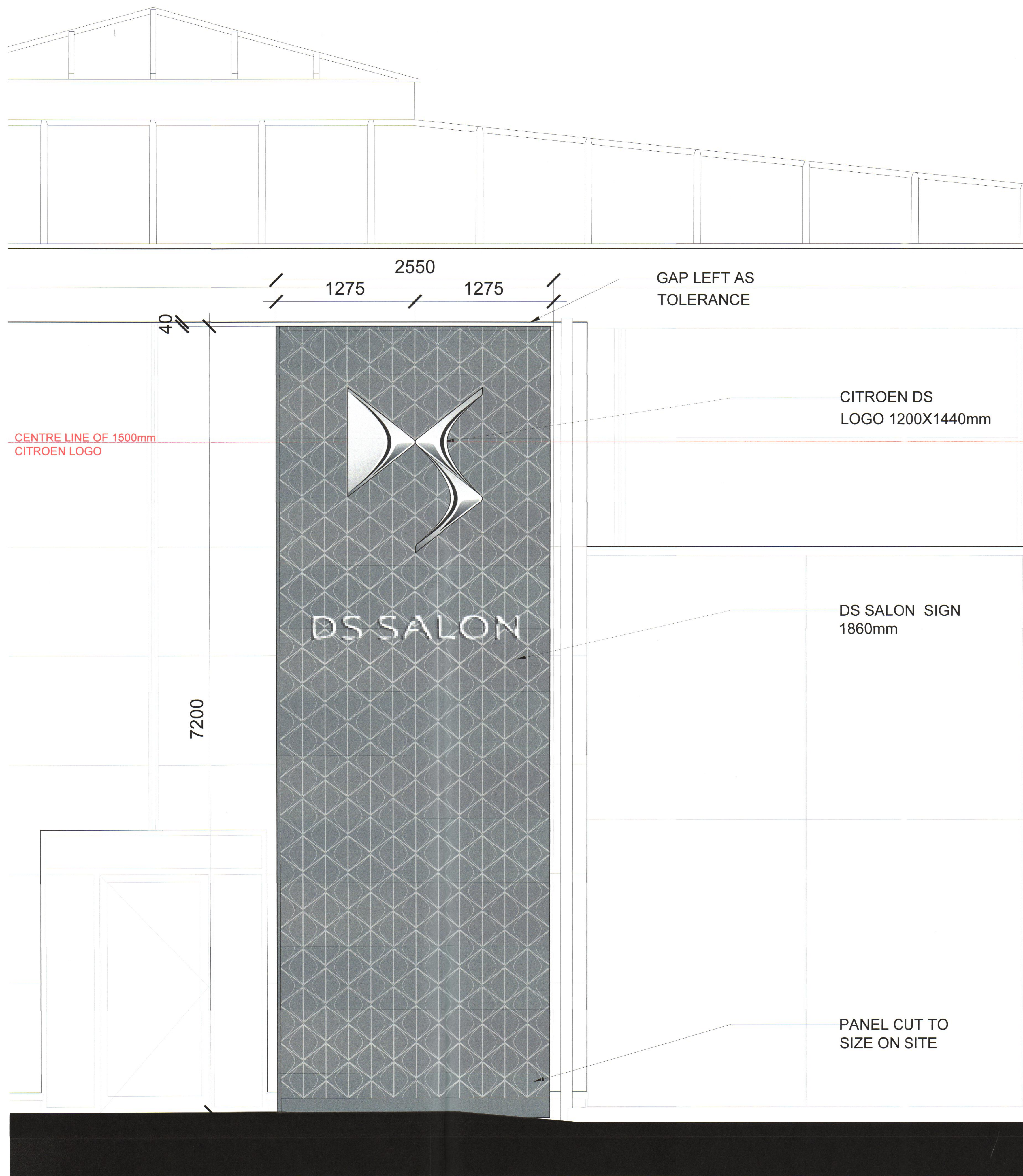
1 TOTEM ELEVATION Scale: 1:20
