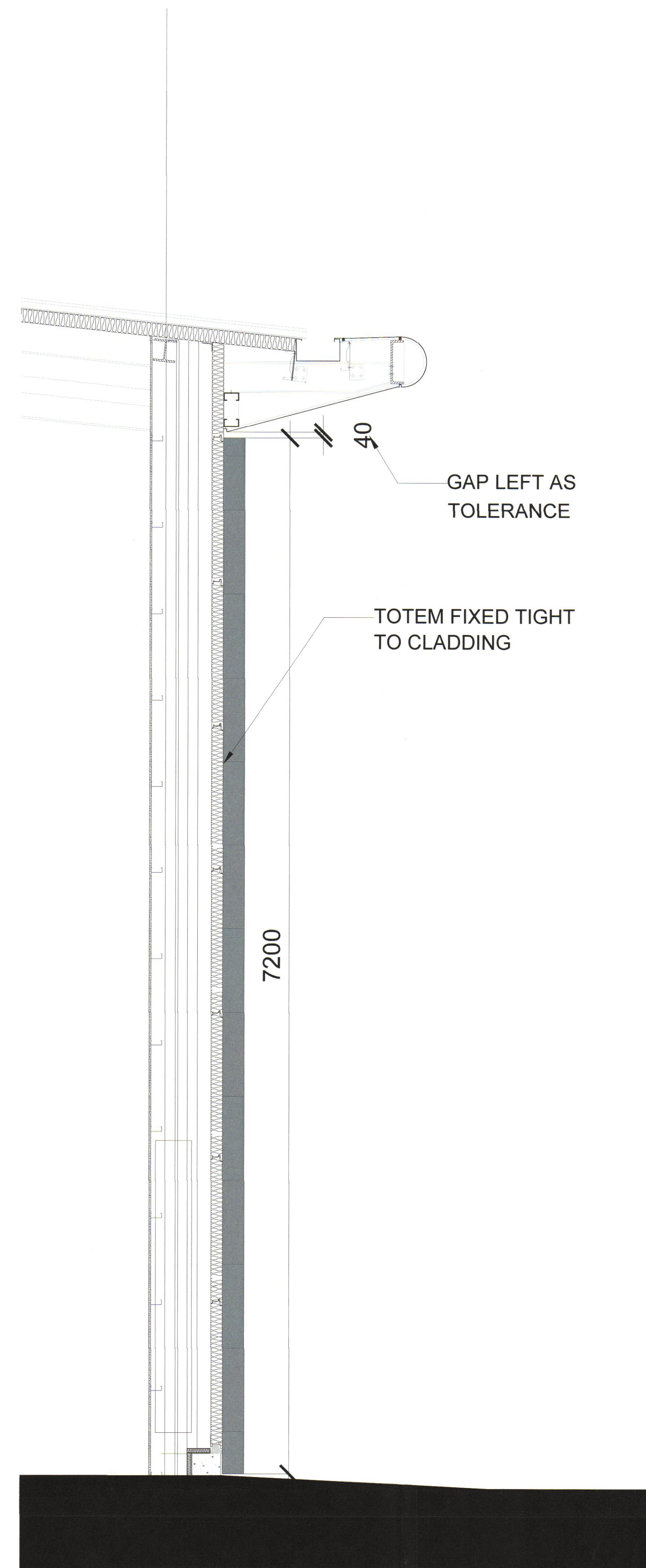
2 TOTEM SECTION Scale: 1:20
