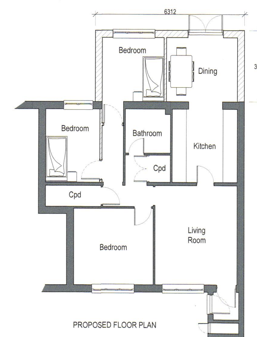
PLAN 1:100
